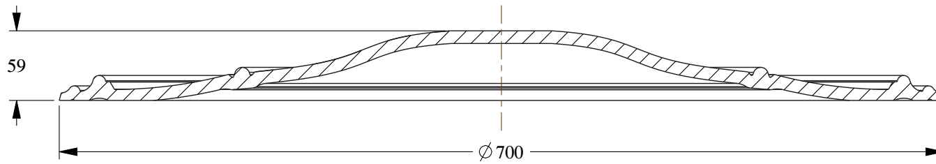
SECTION A-A
