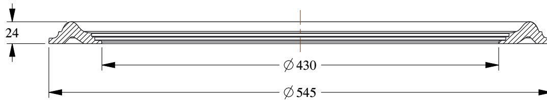
SECTION A-A
