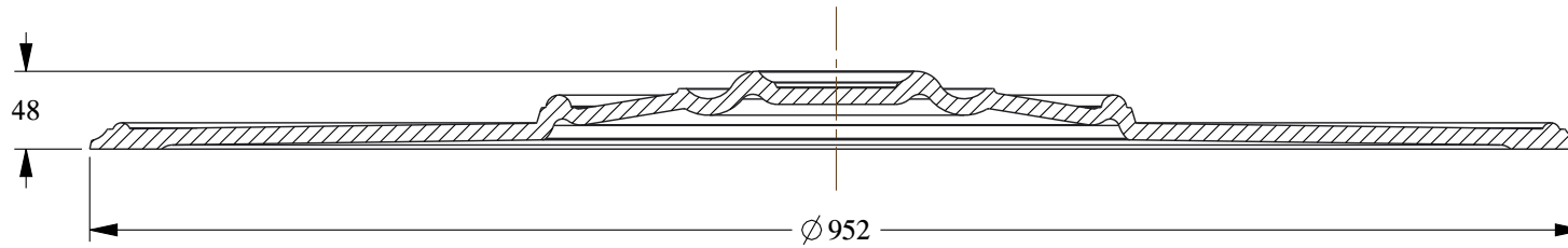
SECTION A-A
