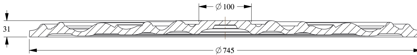
SECTION A-A
