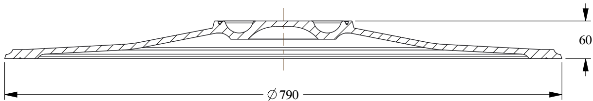
SECTION A-A
