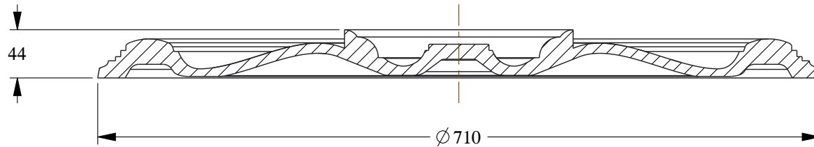
SECTION A-A
