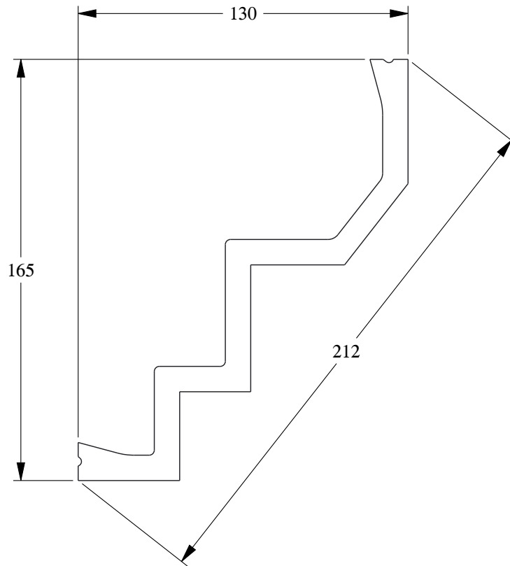
SCALE 1:2
